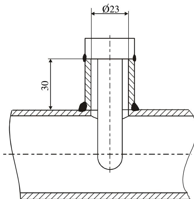
Рисунок 15 - Установка защитной гильзы на трубопроводе при D_n = 50 мм
