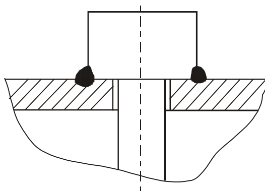
Рисунок 16 - Установка защитной гильзы на трубопроводе при D_n > 50 мм
