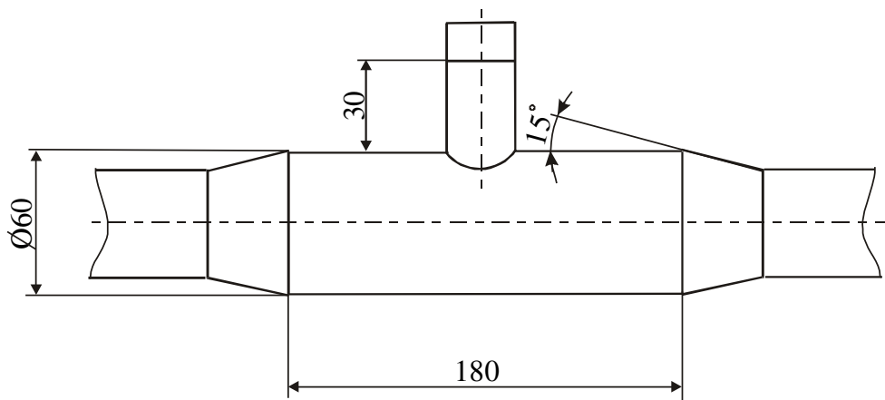
Рисунок 14 - Установка защитной гильзы на трубопроводе при D_n < 50 мм
